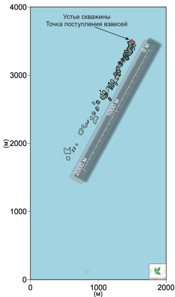
Рисунок 4.8 – Загрязнение водной толщи при вытеснении бурового раствора и шлама при бурении направления 762,0 мм.
