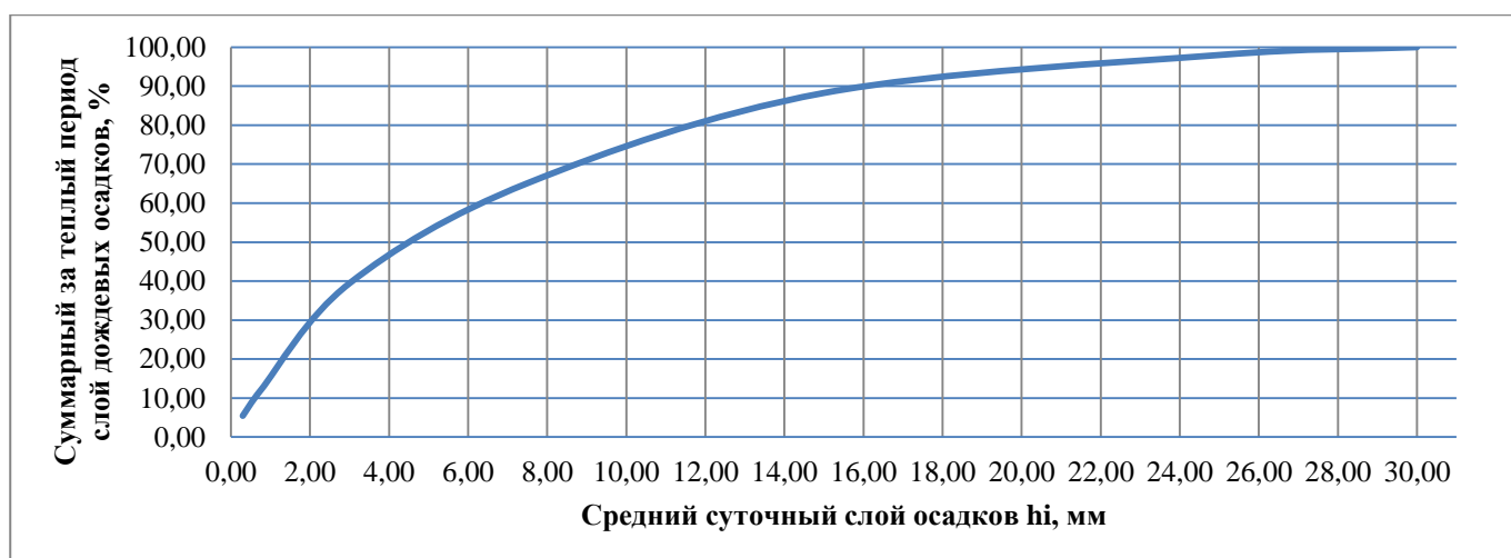
Рисунок 4.6 – График зависимости принимаемой на очистку части осадков от величины максимального суточного слоя дождя
