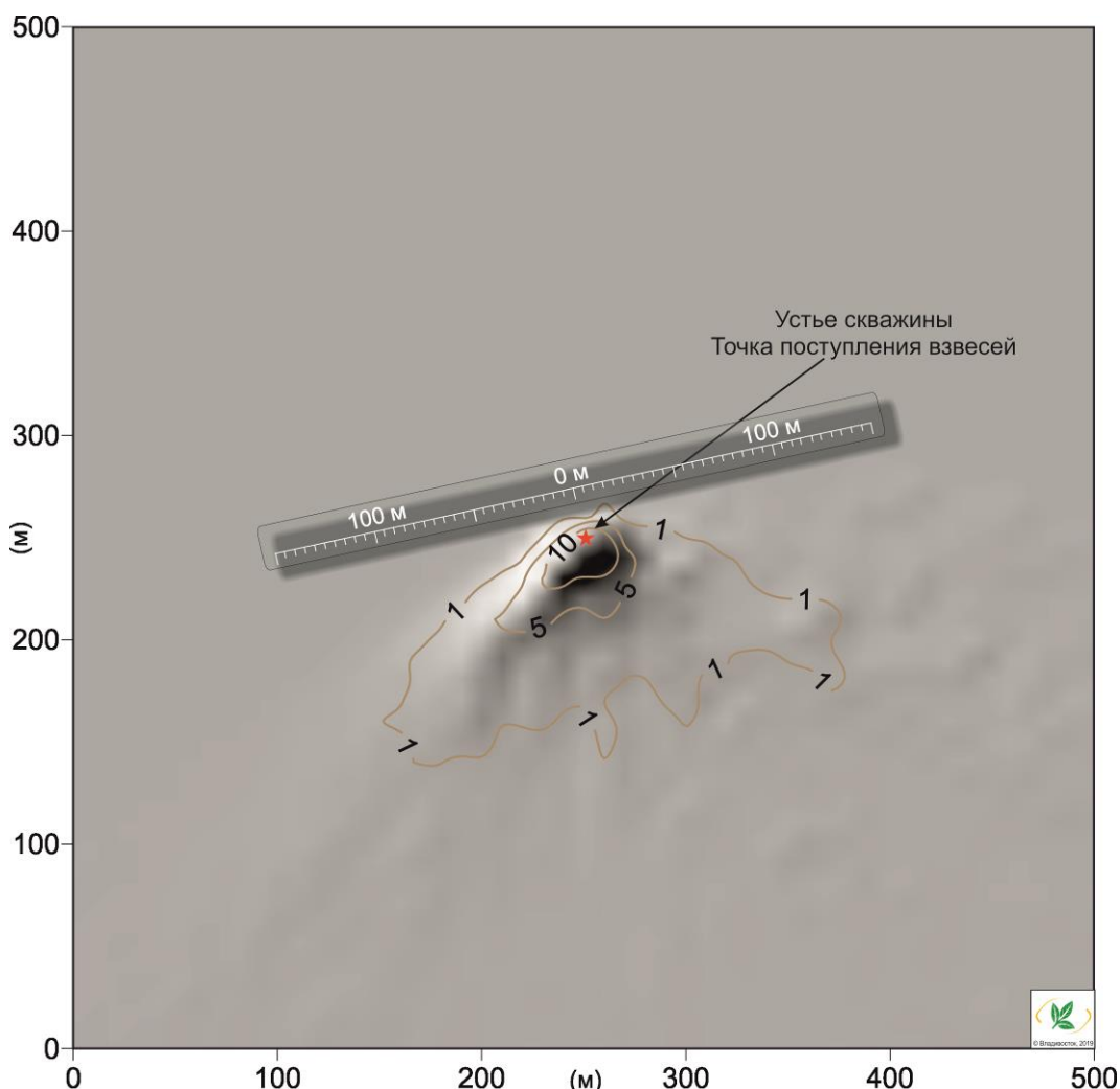
Рисунок 4.9 – Зона осадков на морском дне после окончания вытеснения бурового раствора и шлама
